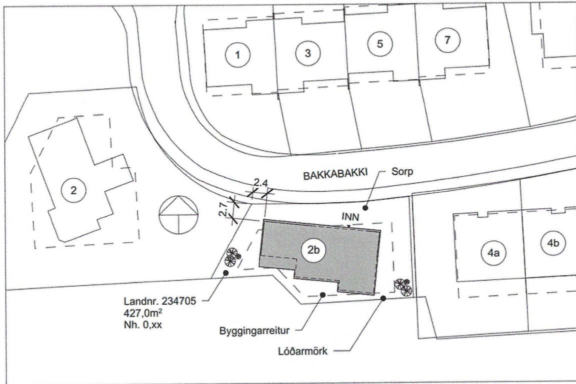
① Afstöðumynd 1 : 500
